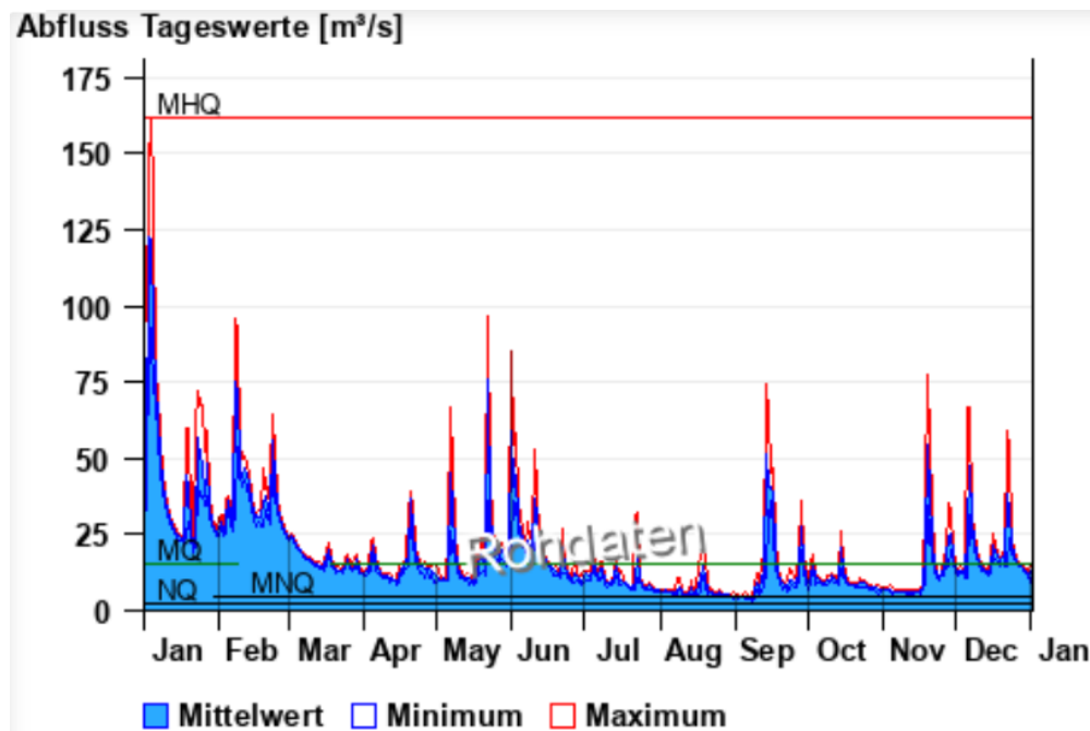
Abbildung 28: Abflussmenge der Ilz
