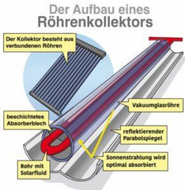
Abbildung 27: Aufbau eines Röhrenkollektors
